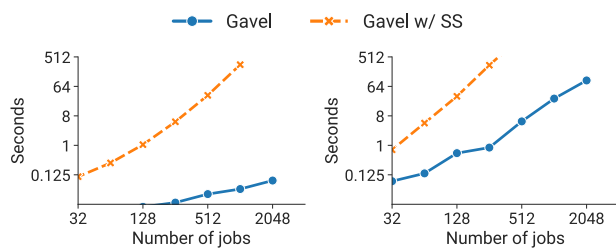
(a) LAS. (b) Hierarchical.
